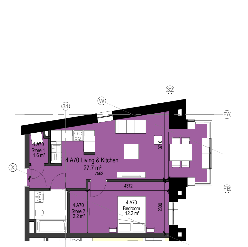
1 1 Bed Type 1I 1 : 100
