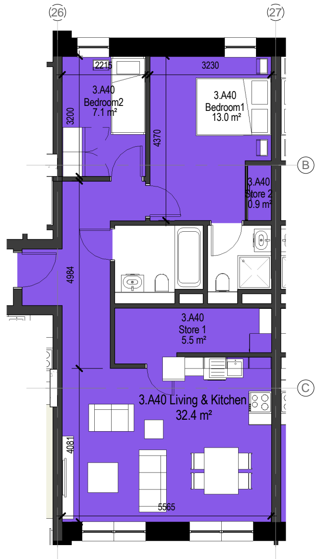
7 2 Bed Type 2.3D 1 : 100
