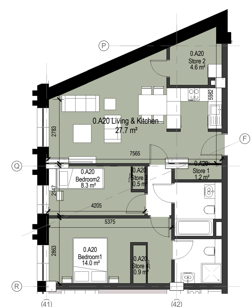
4 2 Bed Type 2.3A 1 : 100
