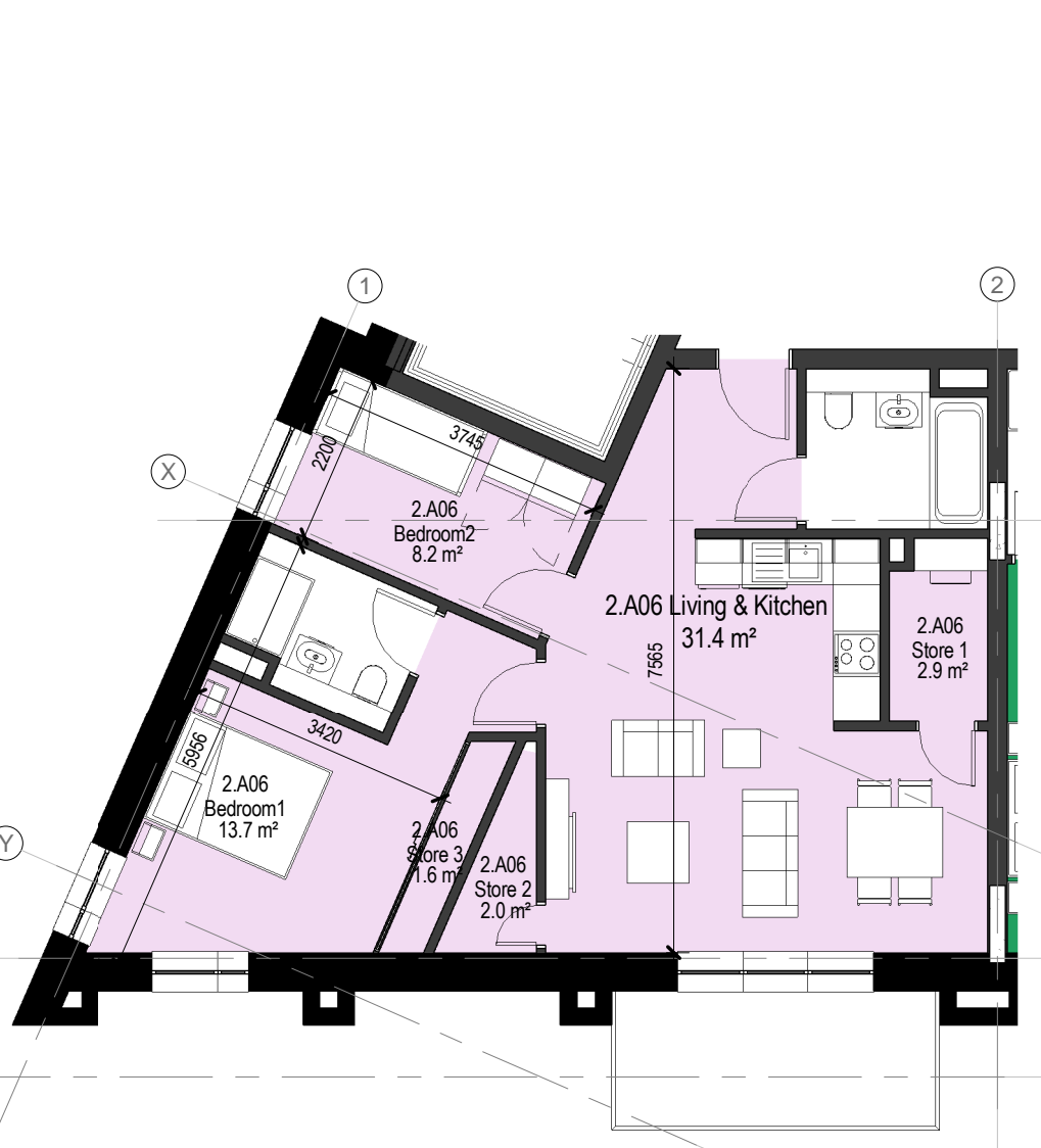
6 2 Bed Type 2.3C 1 : 100
